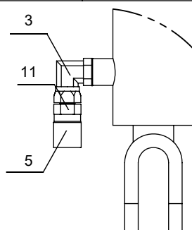
DÉTAIL E ECHELLE 1 : 5
