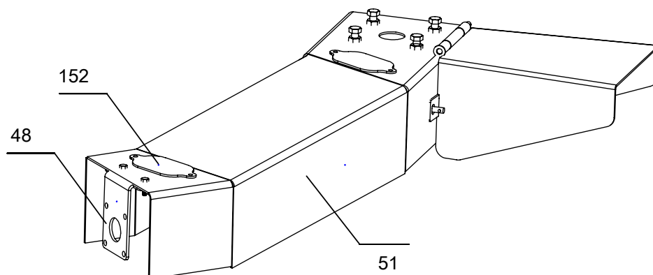
COUVERT DU PTO
