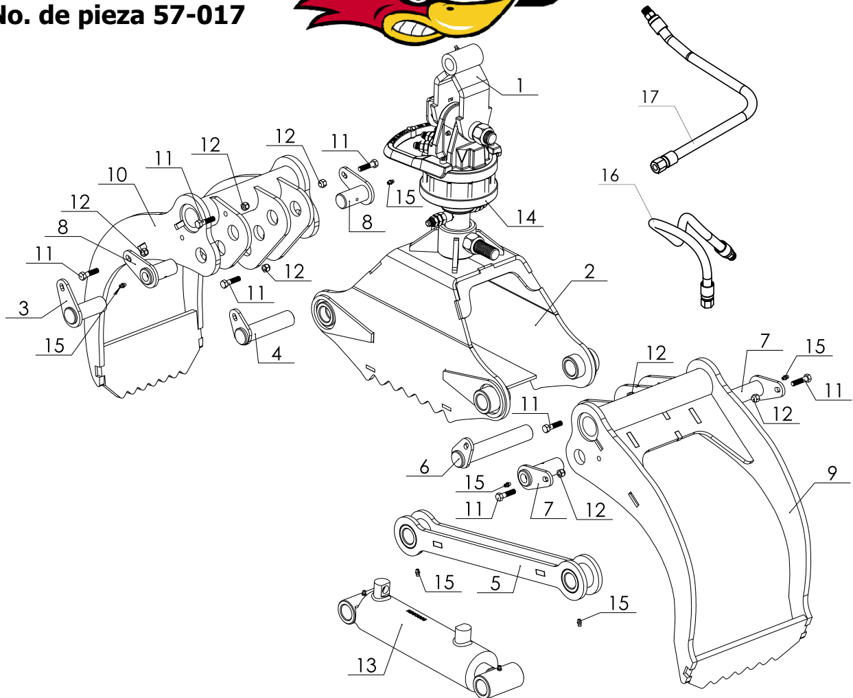
LISTA DE PIEZAS- CONJUNTO DE GARRA DE 42", NO. DE PIEZA 57-017
