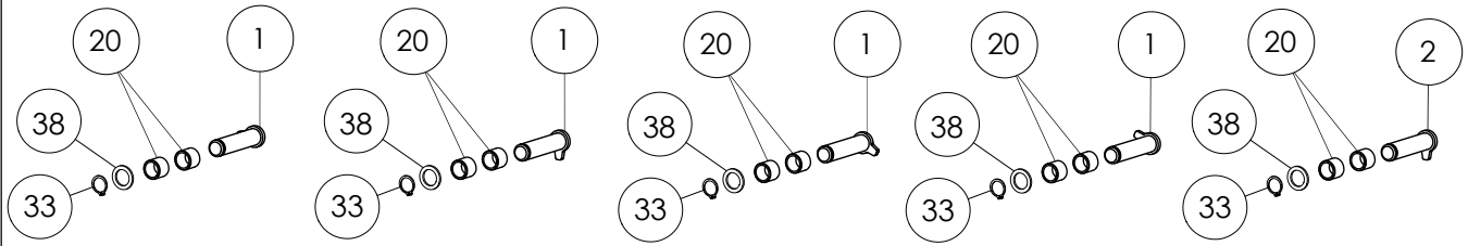
DÉTAIL A ECHELLE 1 : 10
