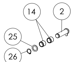
DETALLE E ESCALA 1 : 10
