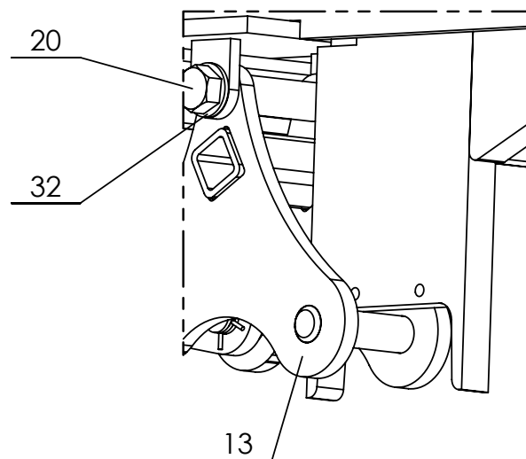
DÉTAIL A ECHELLE 1 : 4
