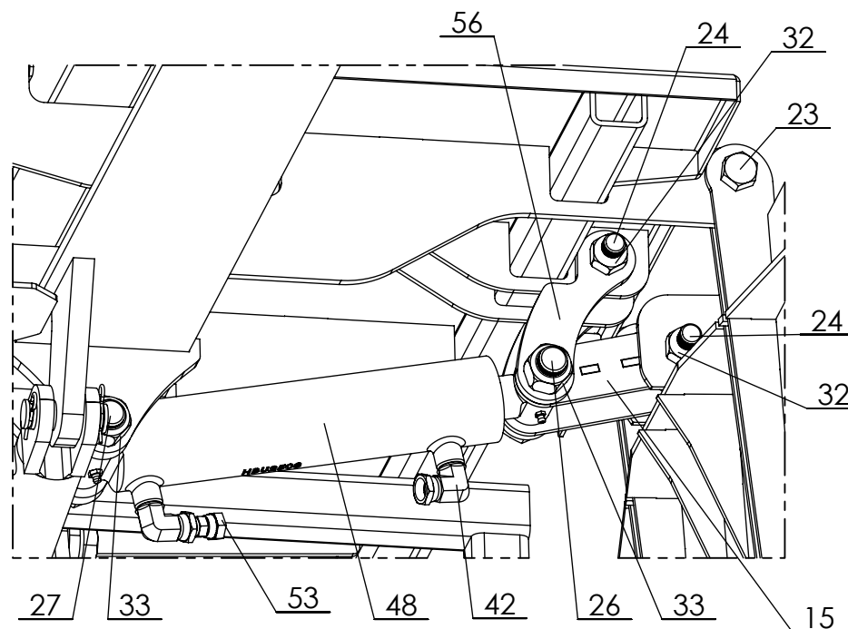
DÉTAIL B ECHELLE 1 : 4
