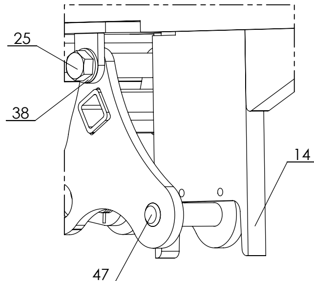
DÉTAIL A ECHELLE 1 : 4
