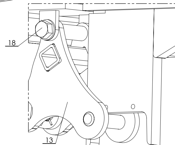
DÉTAIL B ECHELLE 1 : 5
