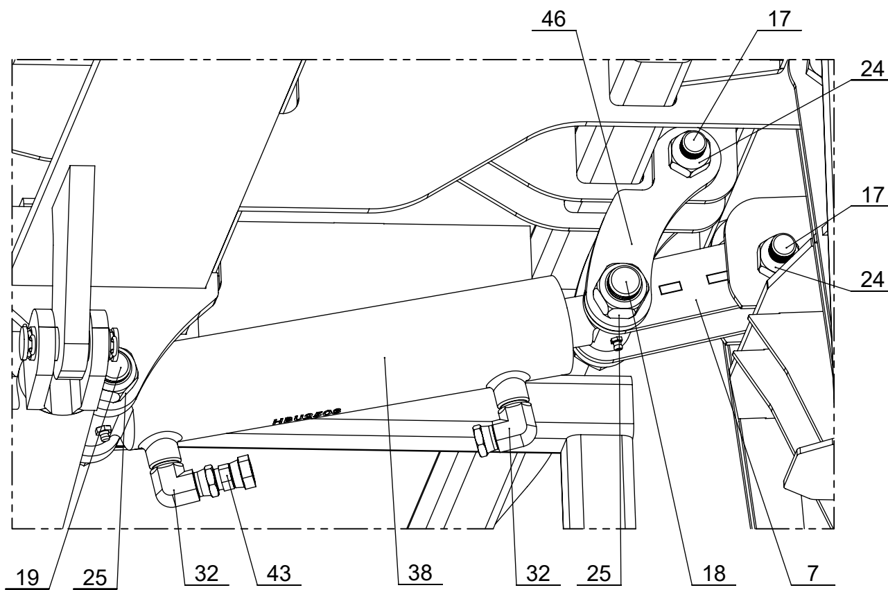
DÉTAIL B ECHELLE 1 : 4
