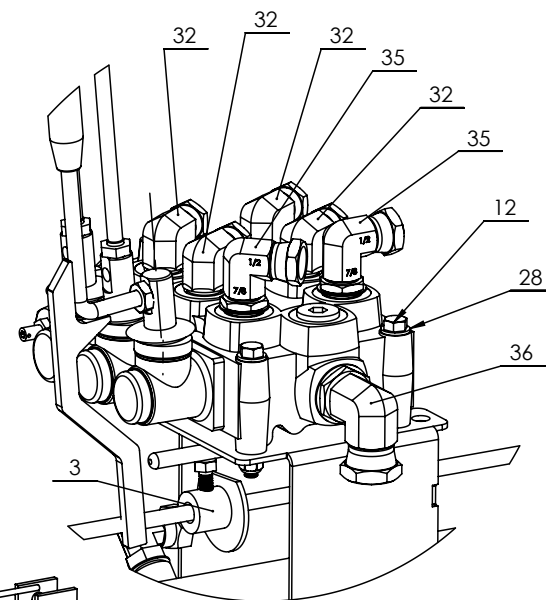
DÉTAIL A ECHELLE 1 : 4
