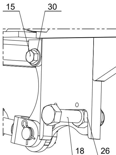
DÉTAIL A ECHELLE 1 : 4
