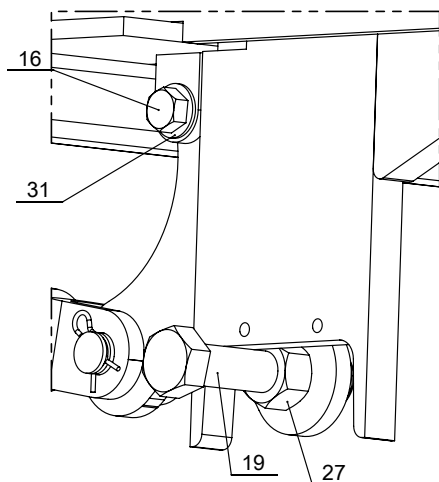
DÉTAIL A ECHELLE 1 : 4
