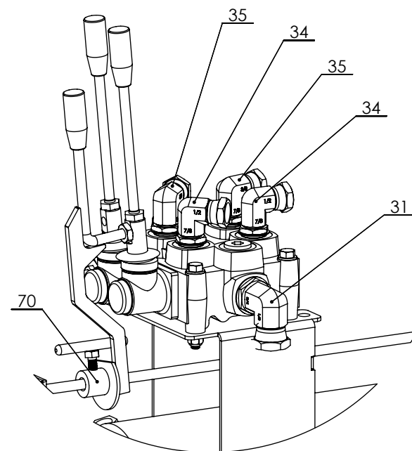
DÉTAIL B ECHELLE 1 : 5
