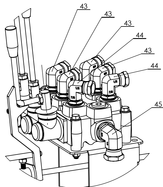
DÉTAIL A ECHELLE 1 : 4
