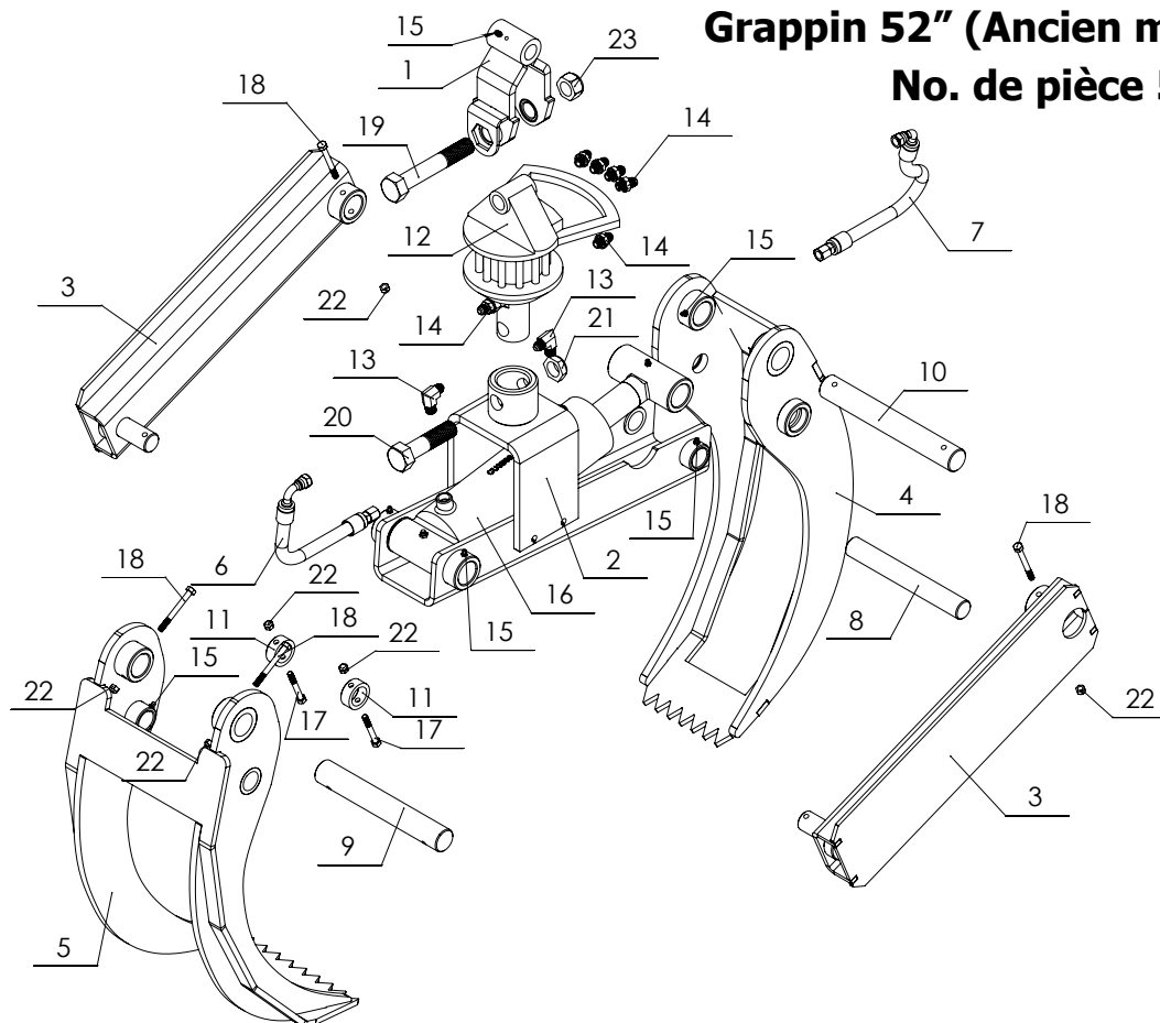
LISTE DES PIÈCES - ASSEMBLAGE GRAPPIN DE 52", NO. DE PIÈCE 57-004
