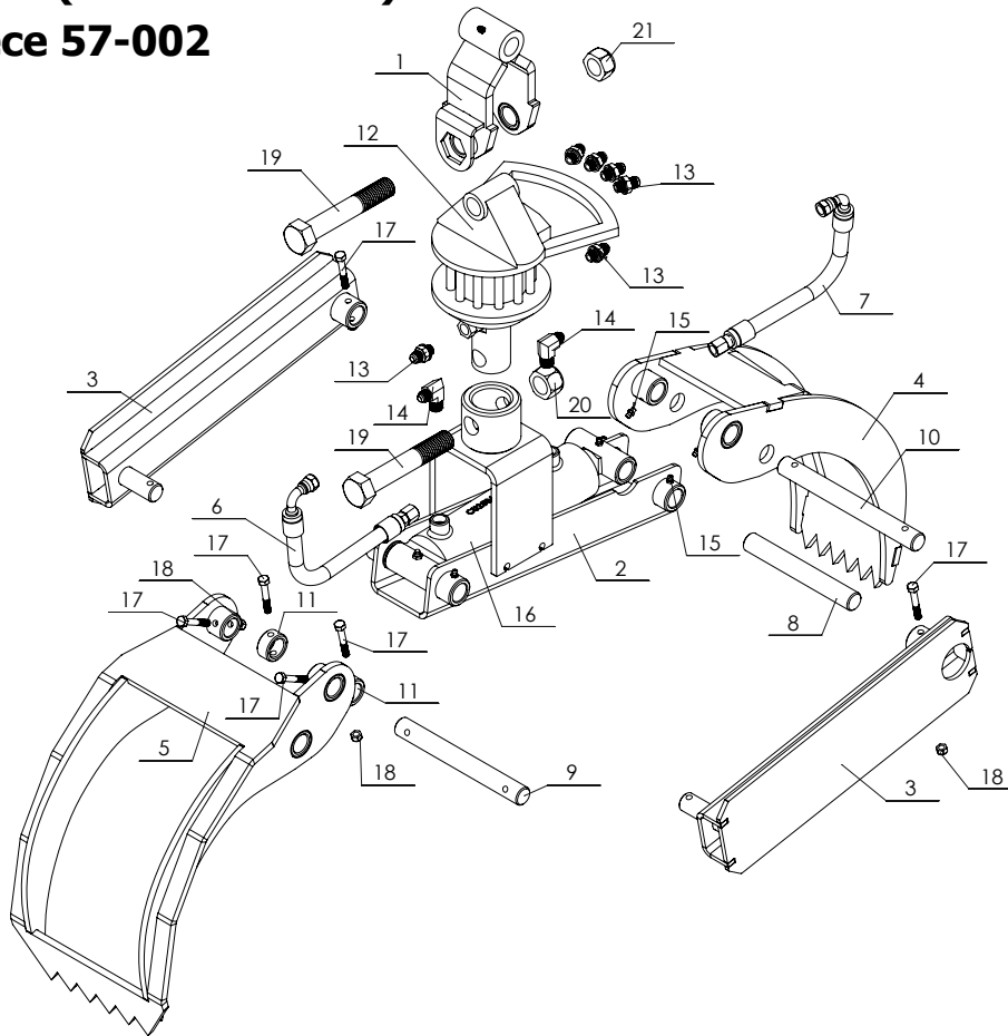
Liste de Pièces - Grappin 36" No. de pièce 57-002
