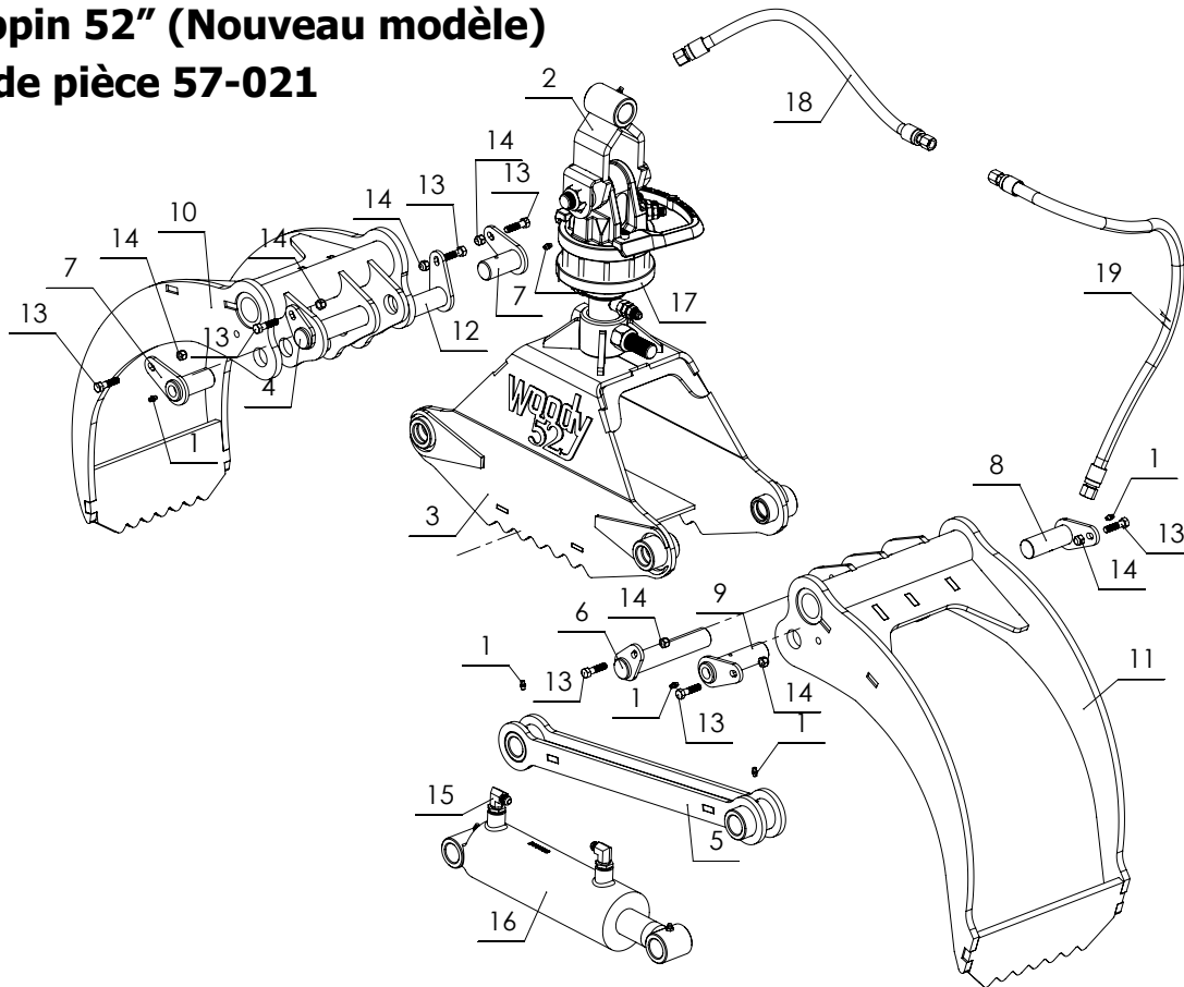
LISTE DES PIÈCES - ASSEMBLAGE GRAPPIN DE 52", NO. DE PIÈCE 57-021
