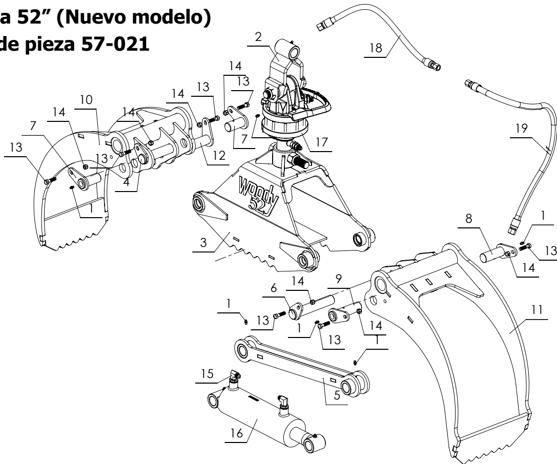
LISTA DE PIEZAS - CONJUNTO DE GARRA DE 52", NO. DE PIEZA 57-021
