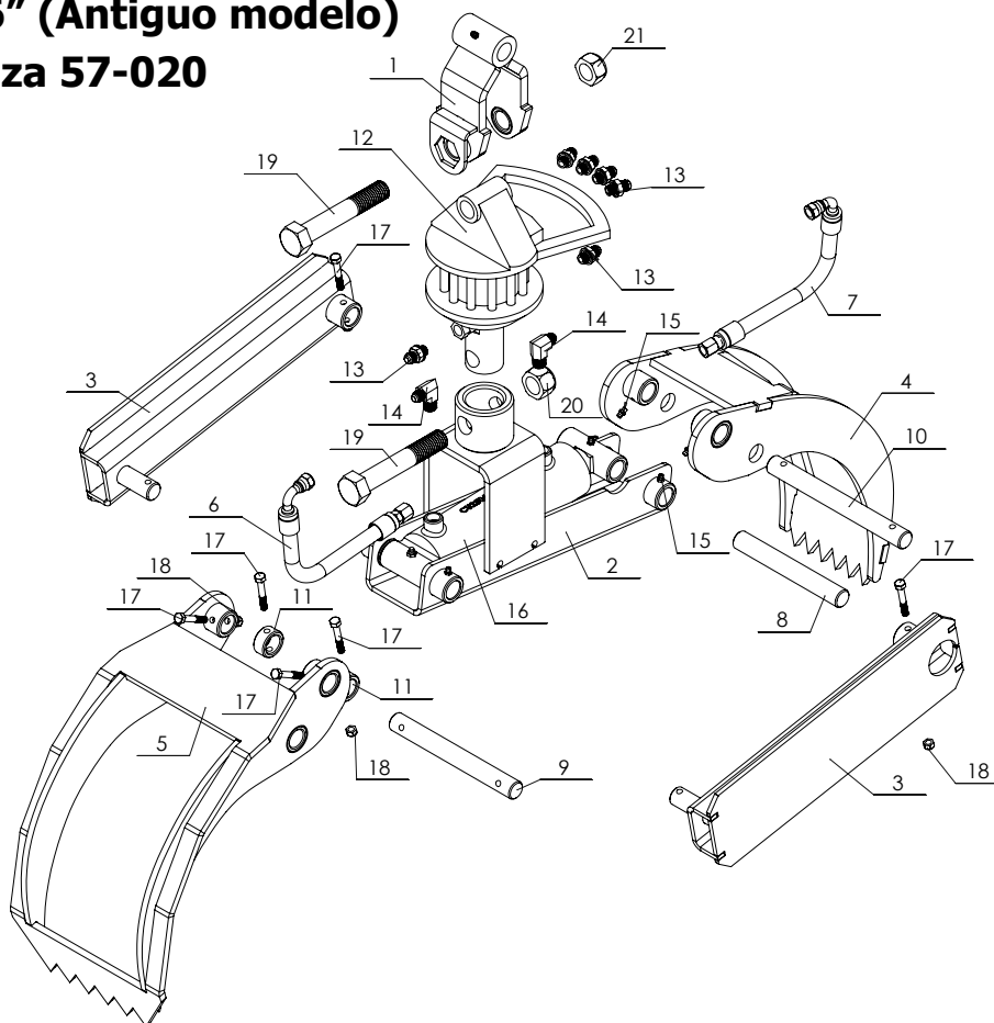
Lista de piezas - Garra de 36" (Antiguo modelo)
