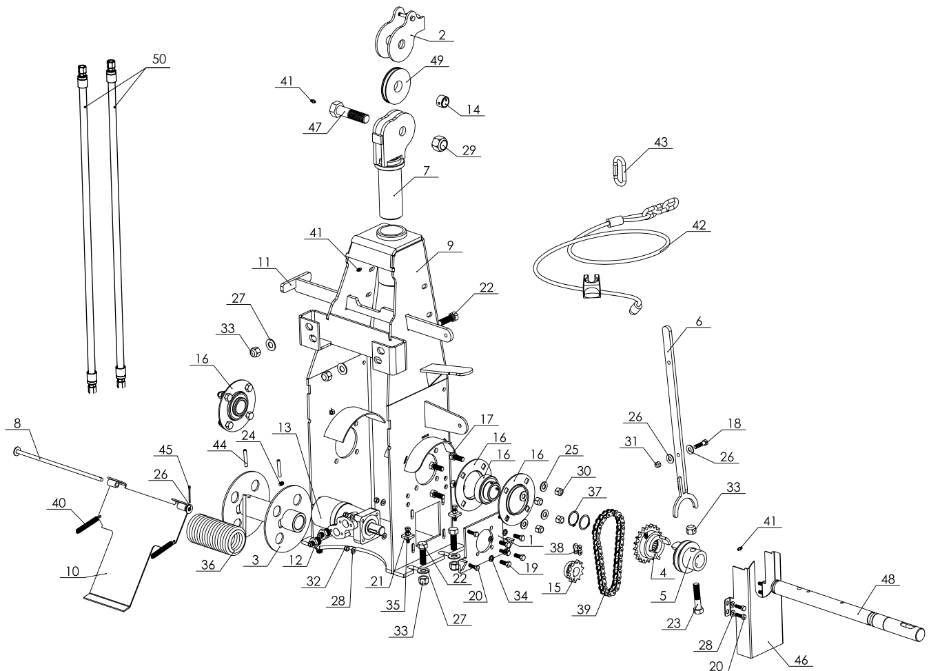
LISTA DE PIEZAS - CONJUNTO CABRESTANTE HIDRÁULICO DE 6000 LB, NO. D EPIEZA 58-007
