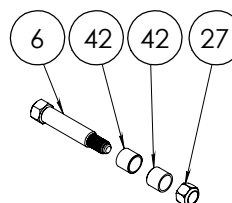
DÉTAIL BA ECHELLE 1:10
